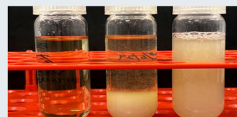
沈殿形成＝リン酸と金属イオン
